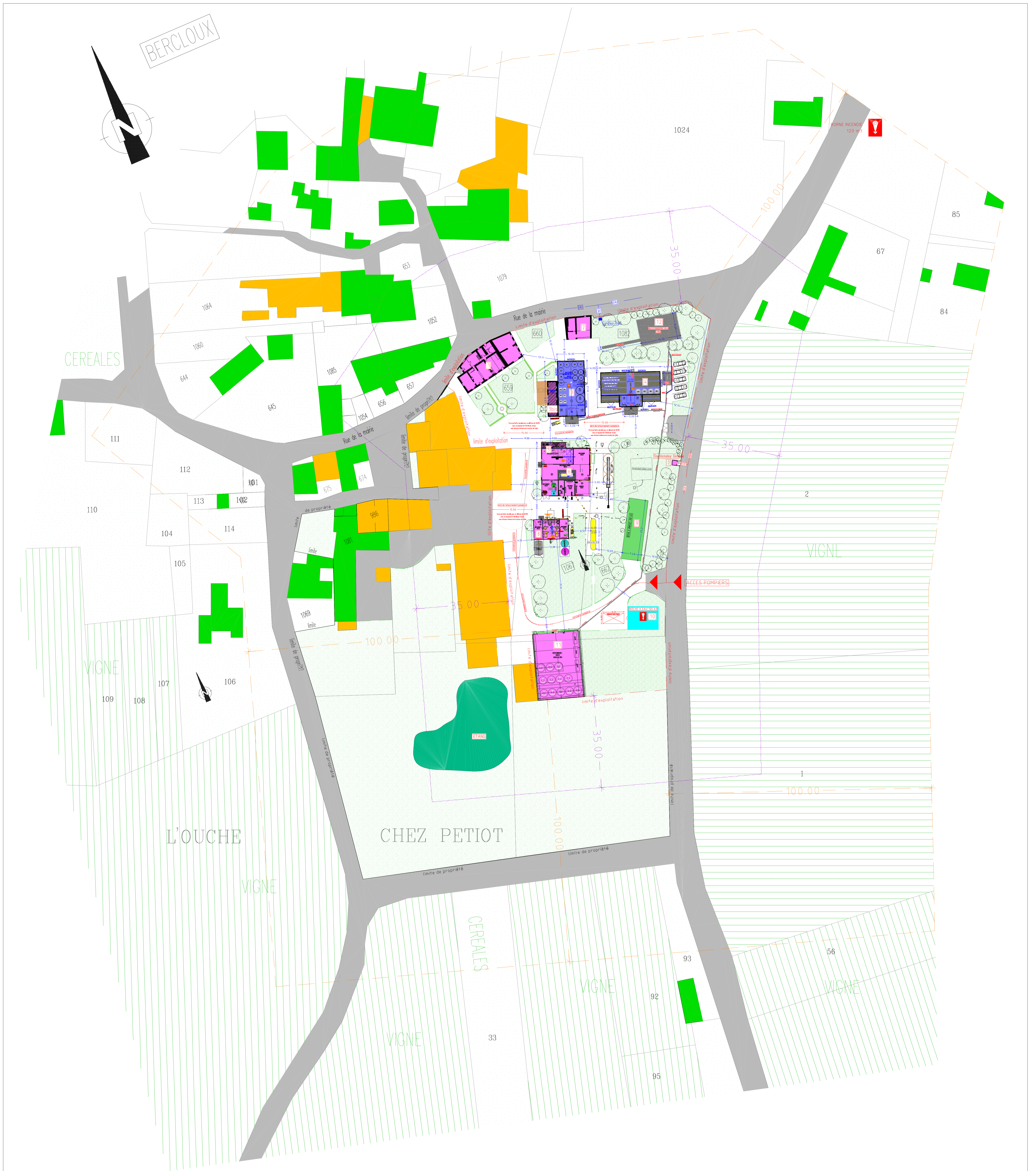
DISTILLERIE DE BERCLOUX PLAN DE MASSE ECHELLE 1/500
